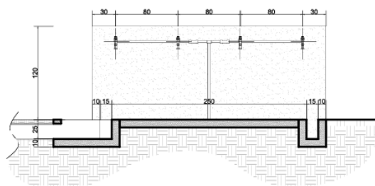
COUPE M-M ESPACE DE PUISAGE
