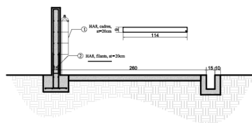
COUPE N-N ESPACE DE PUISAGE
