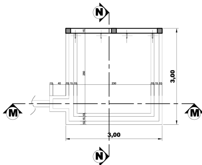
PLAN DE PRINCIPE ESPACE DE PUISAGE
